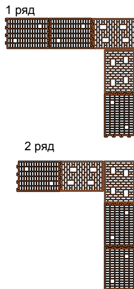
Угол стены
